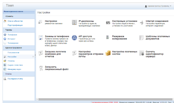
Рис. 1 Вкладка «Настройки»
